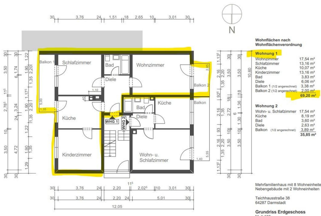
Grundriss
