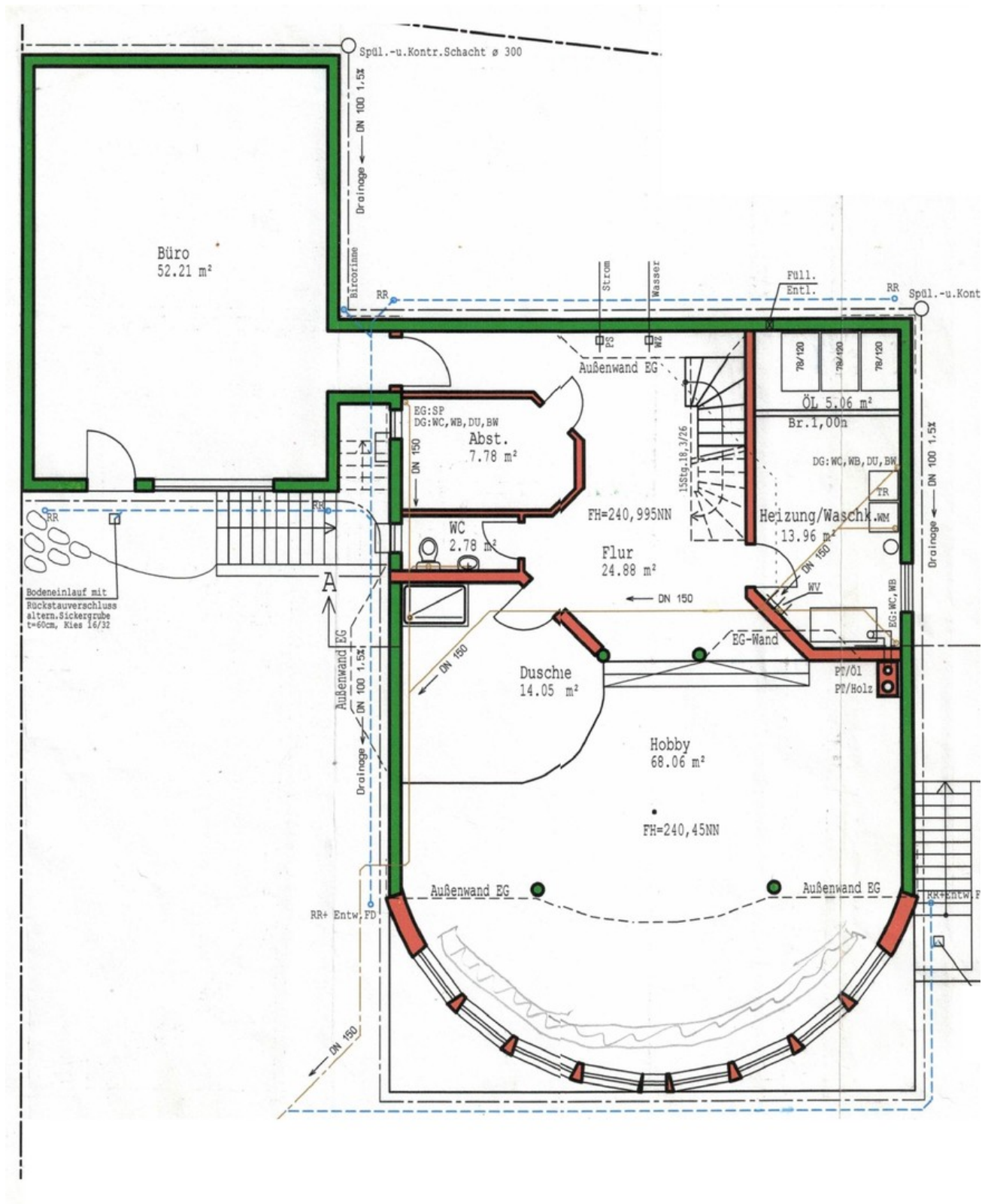
Grundriss UG
