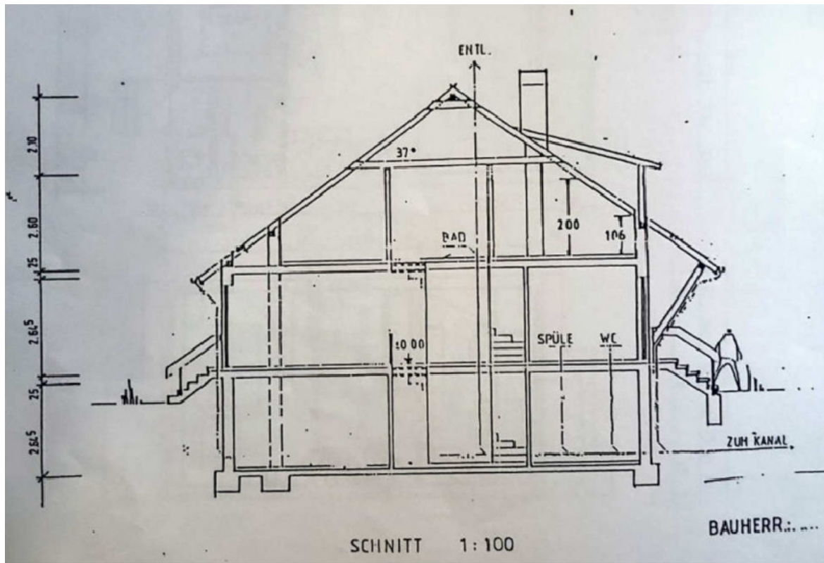
Abbildung 6: Schnitt
