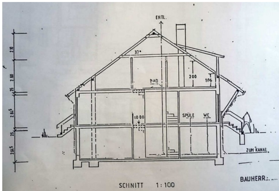
Abbildung 6: Schnitt
