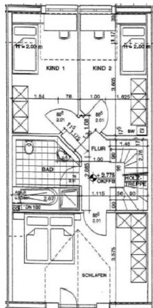
Obergeschoss
