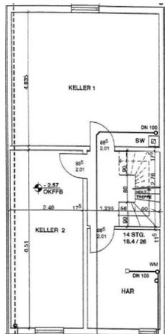
Kellergeschoss
