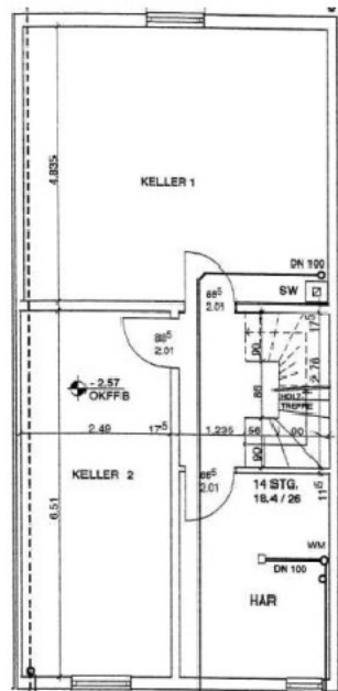
Kellergeschoss
