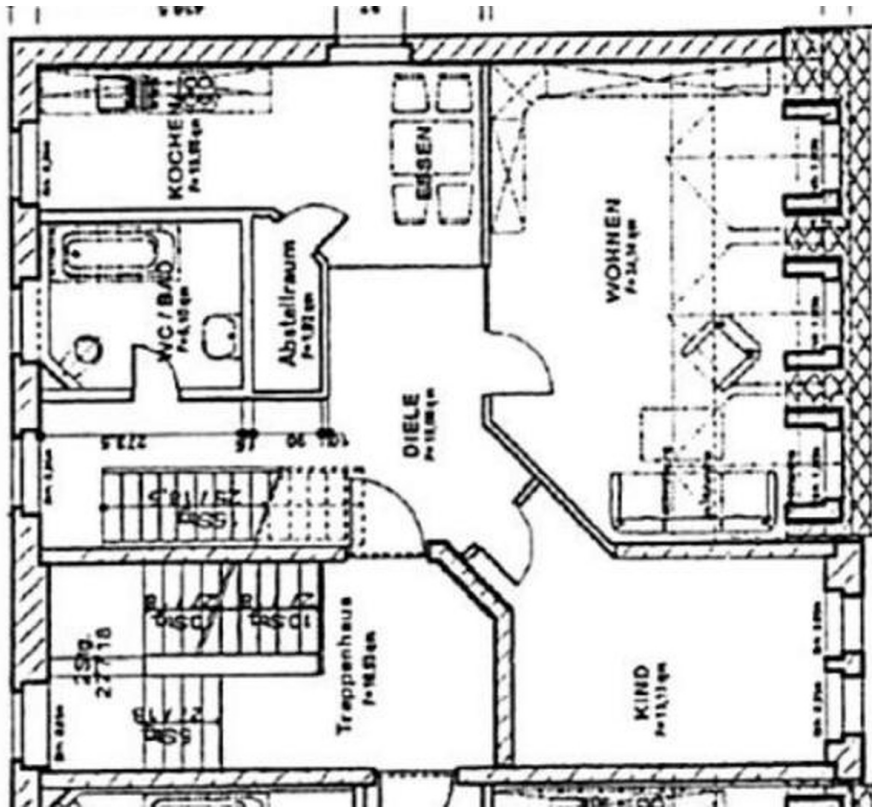
untere Etage
