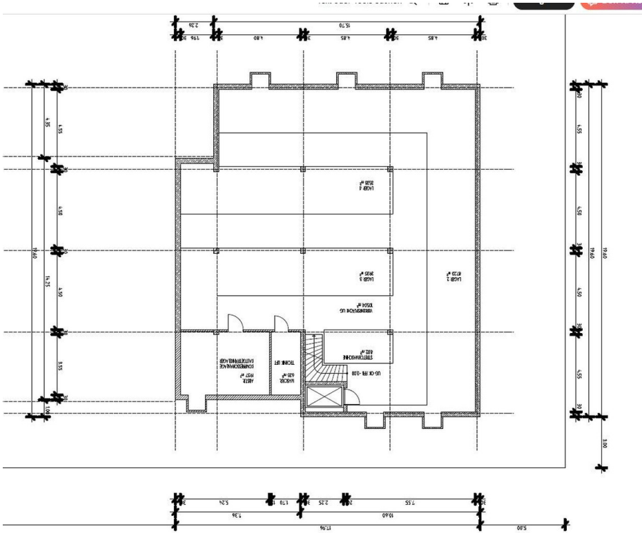
Grundriss Keller
