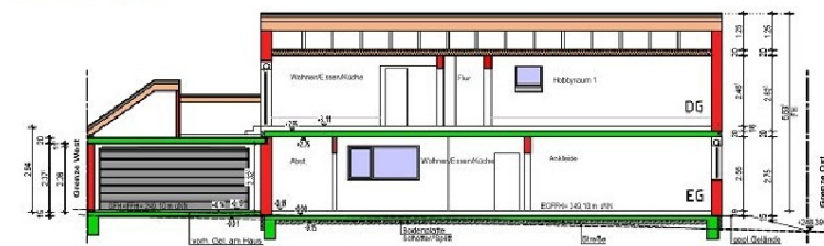
SCHNITT B-B
