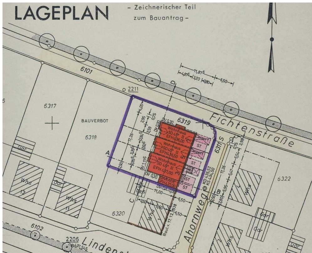
Lageplan
