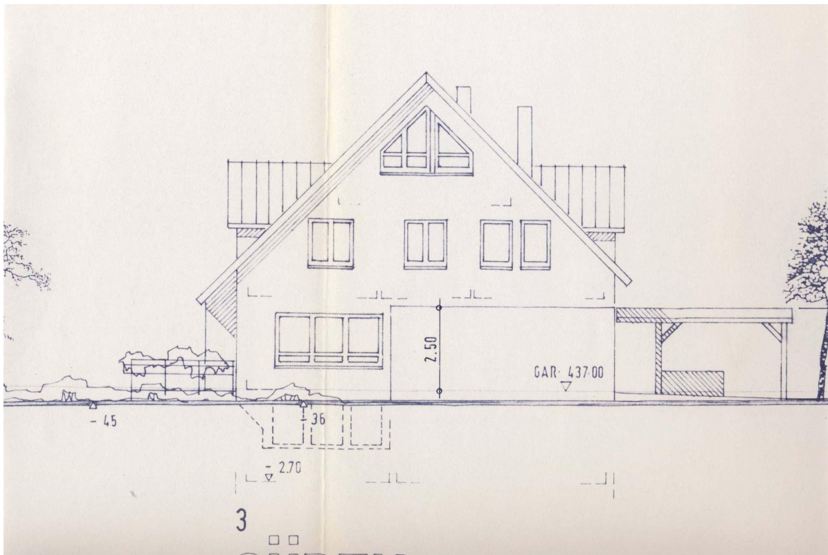
Ansicht Süd
