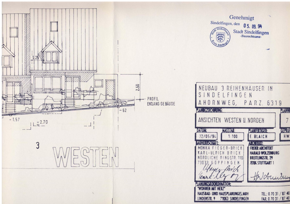
Ansicht West
