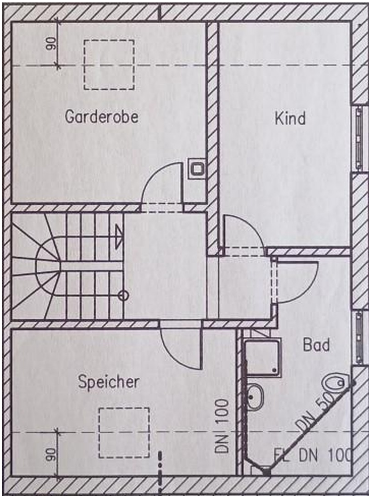
Dachgeschoss
