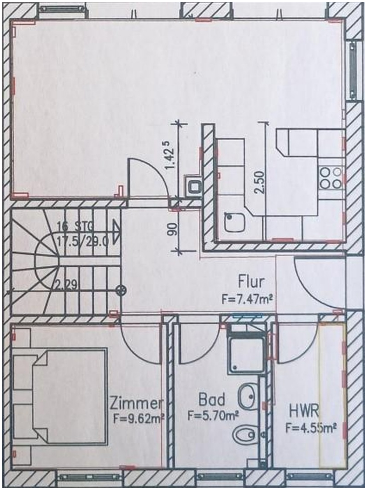
Erdgeschoß
