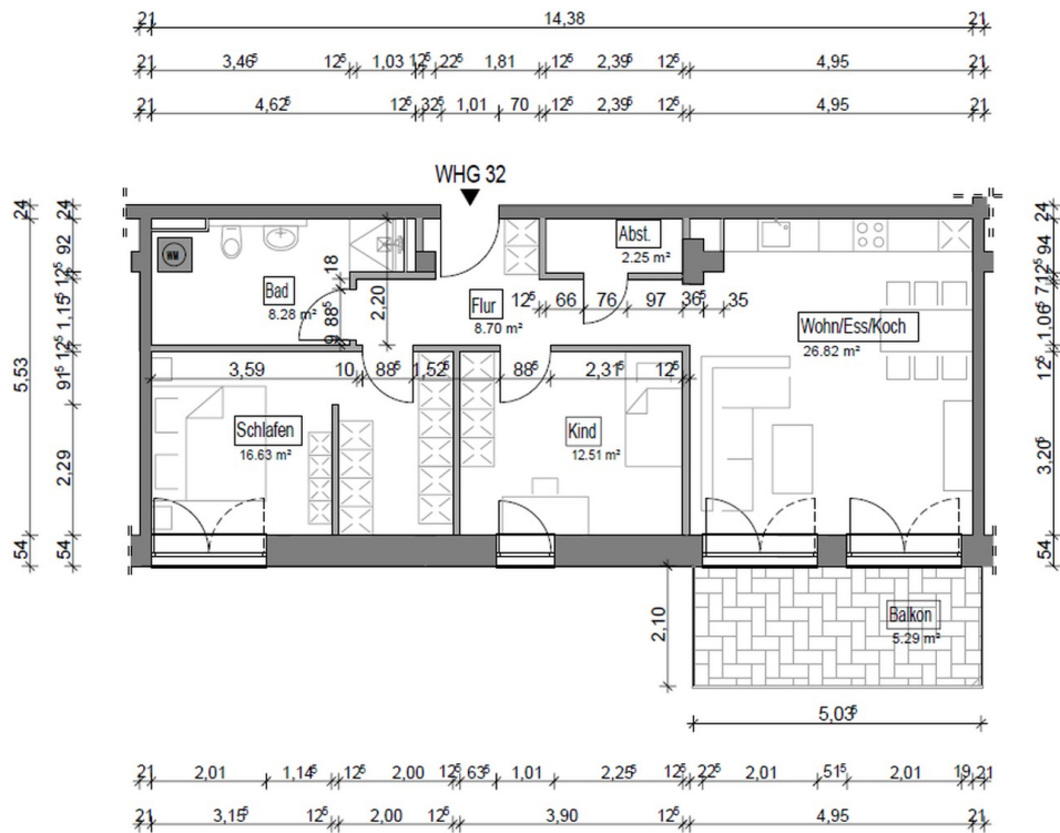
Grundriss
