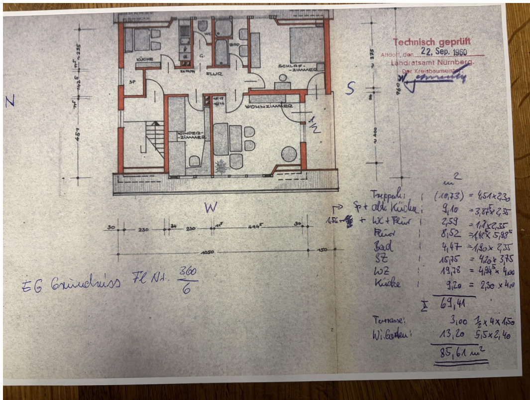
EG Grundriss Bestandsgebäude
