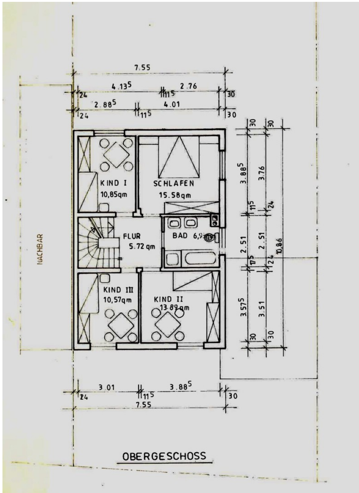
Obergeschoss
