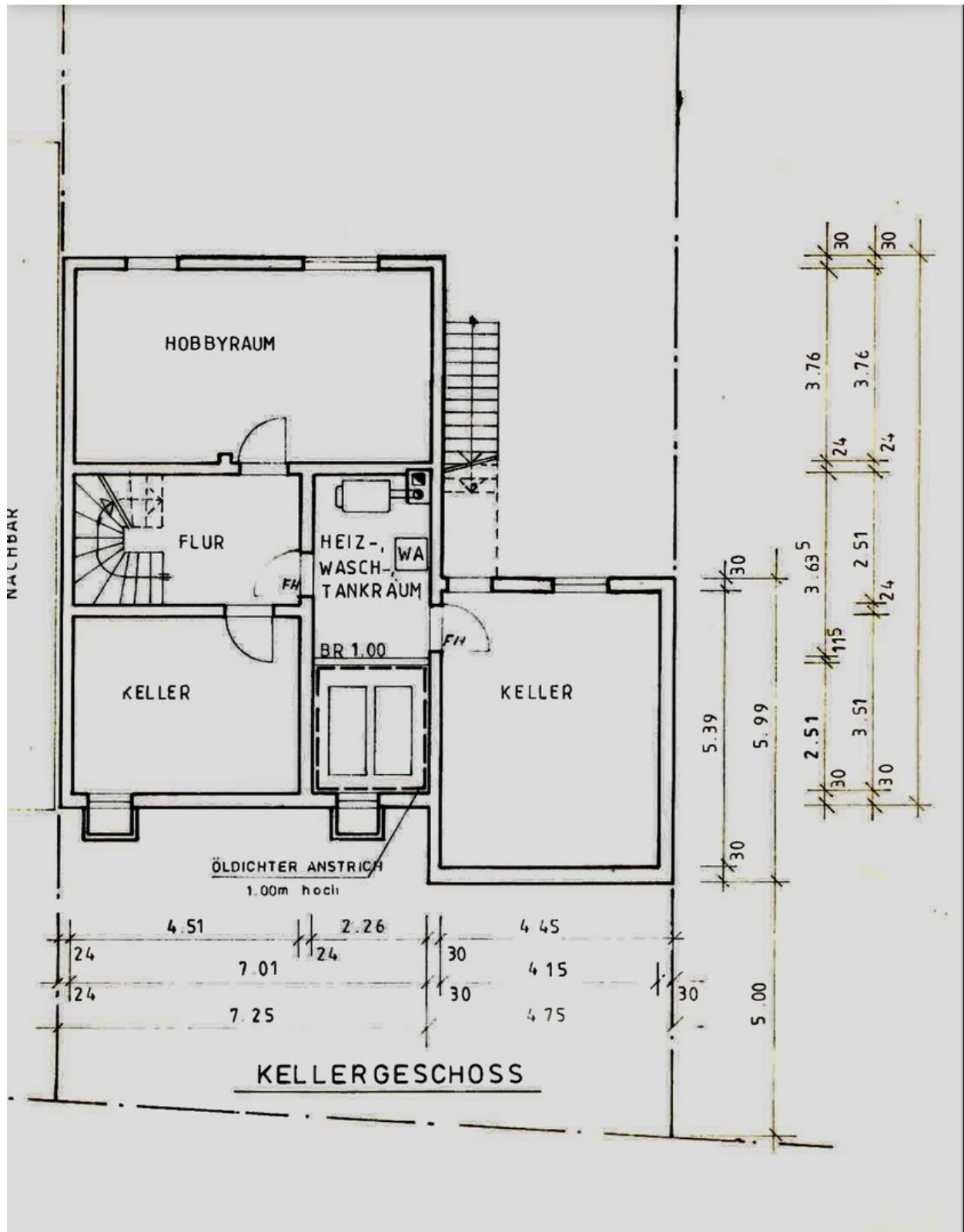
Kellergeschoss
