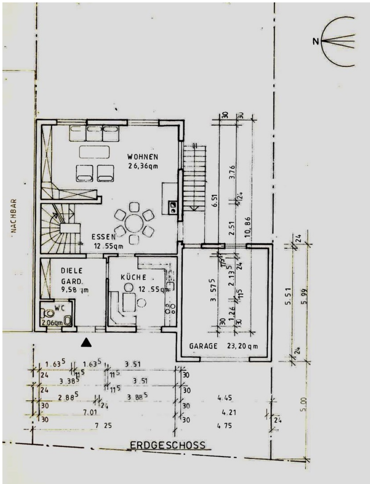
Erdgeschoss
