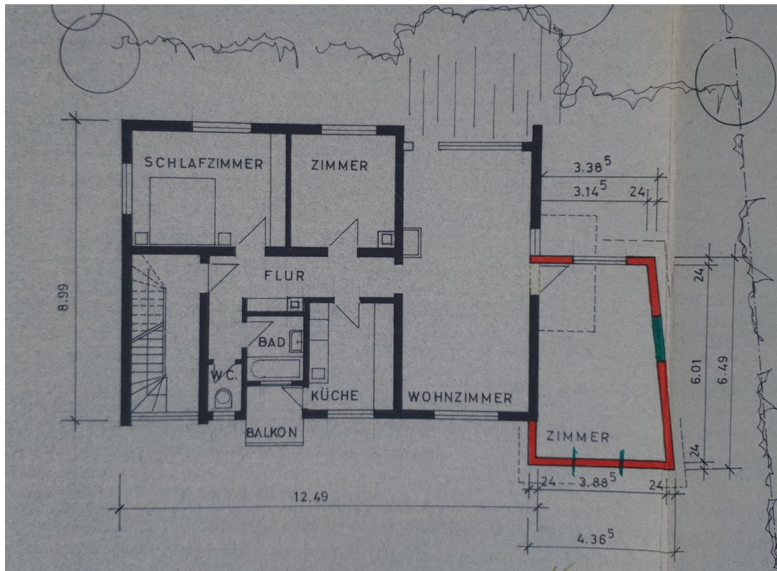
10G Grundriss 1980 mit Anbau
