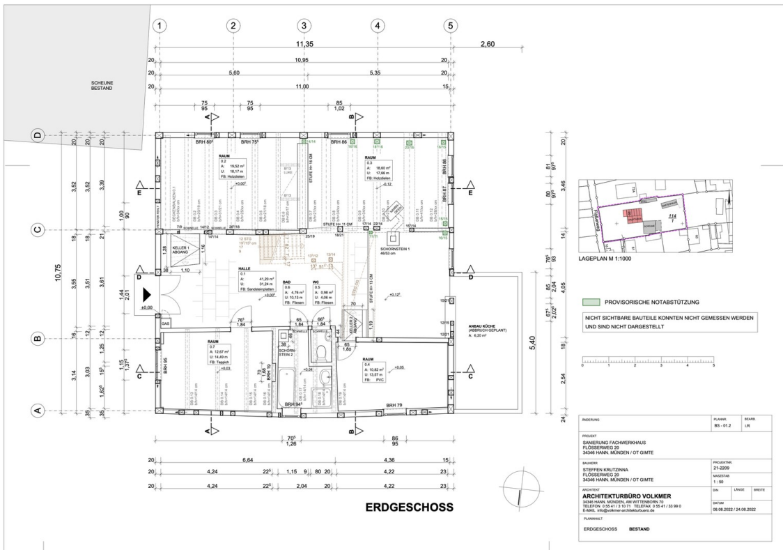
Wohnhaus Erdgeschoss
