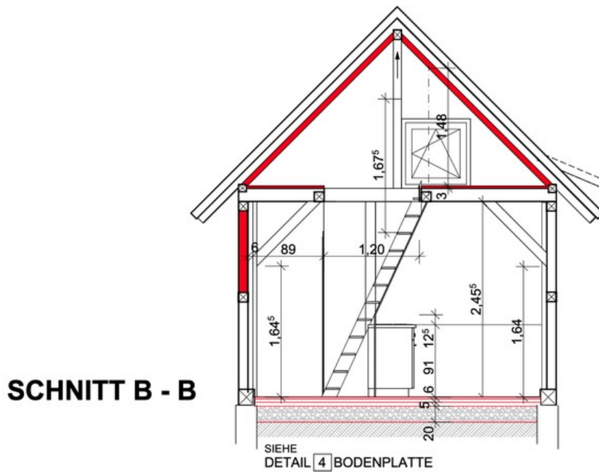
Backhaus Schnitte
