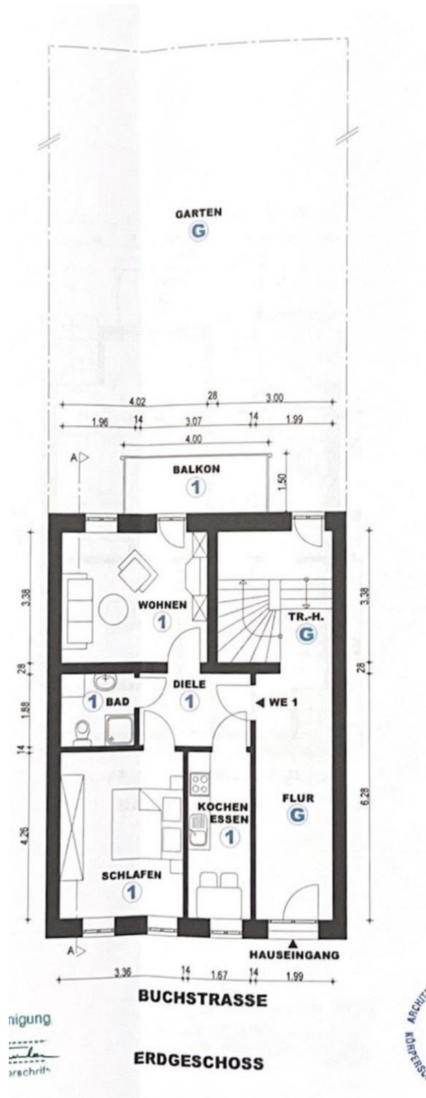
Erdgeschoss
