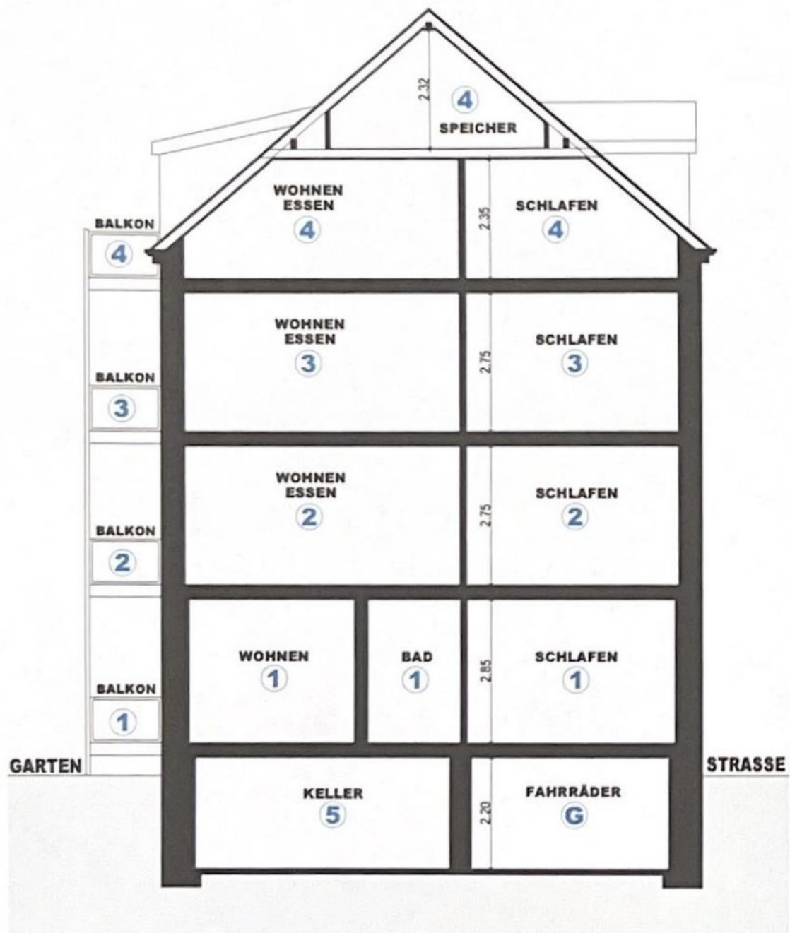
SCHNITT A-A
