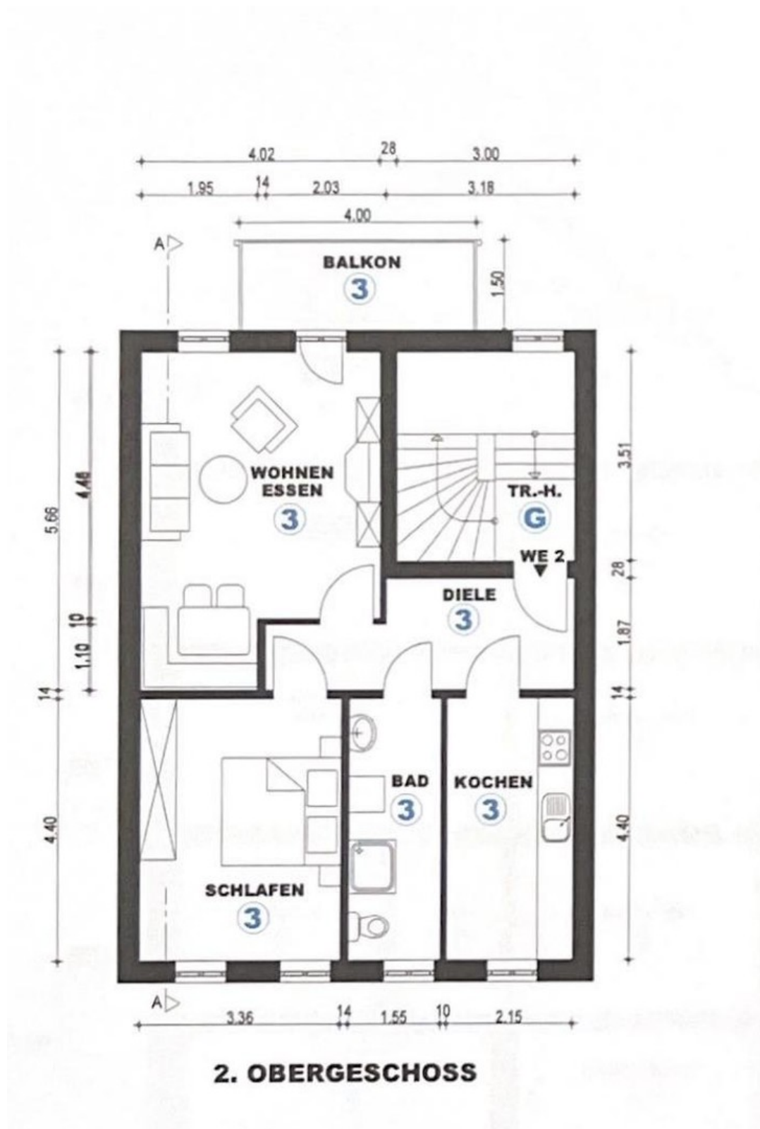
2. Obergeschoss
