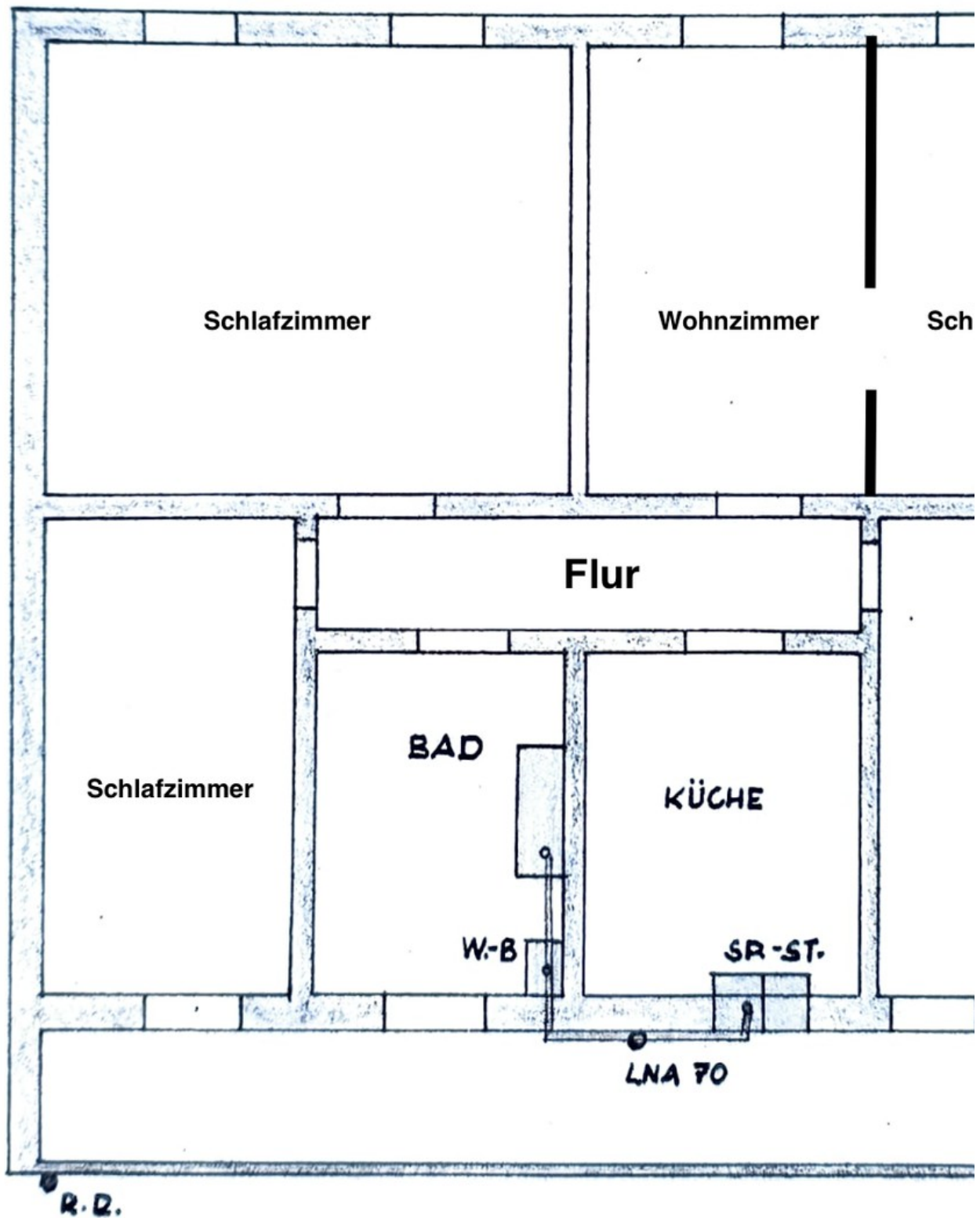
Grundriss
