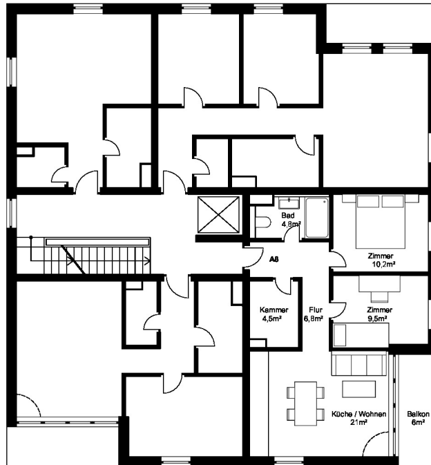
Grundriss 1. Obergeschoss
