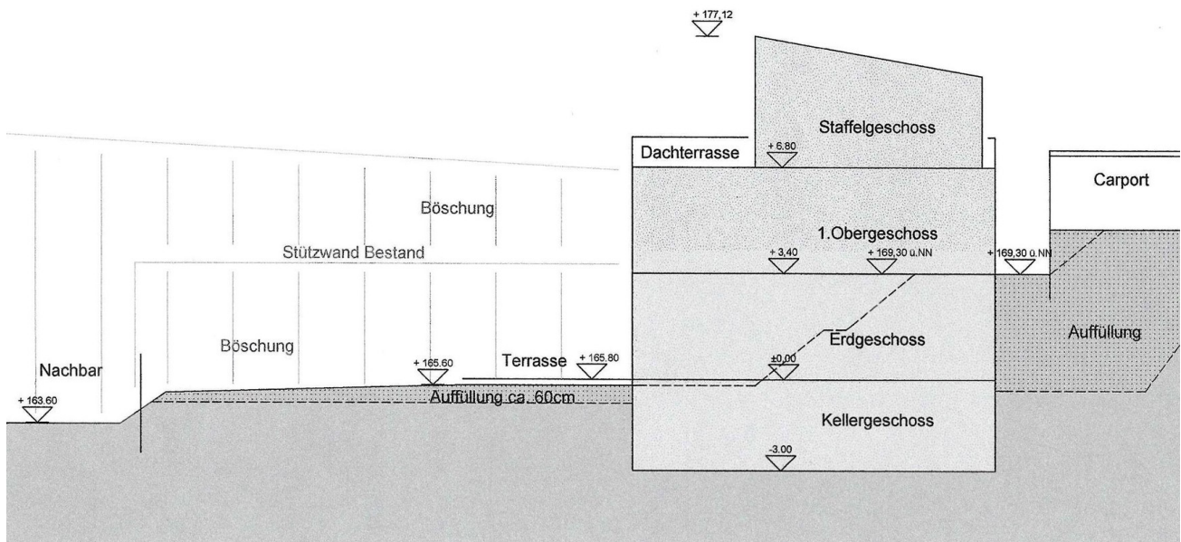
Schnitt A-A
