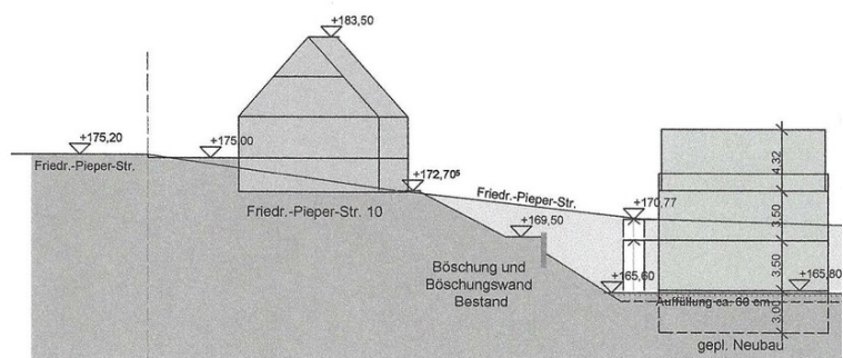
Geländeschnitt Richtung Osten B-B
