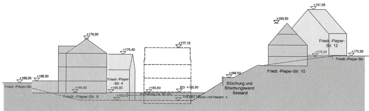
Geländeschnitt Richtung Westen C-C Geländeschnitt
