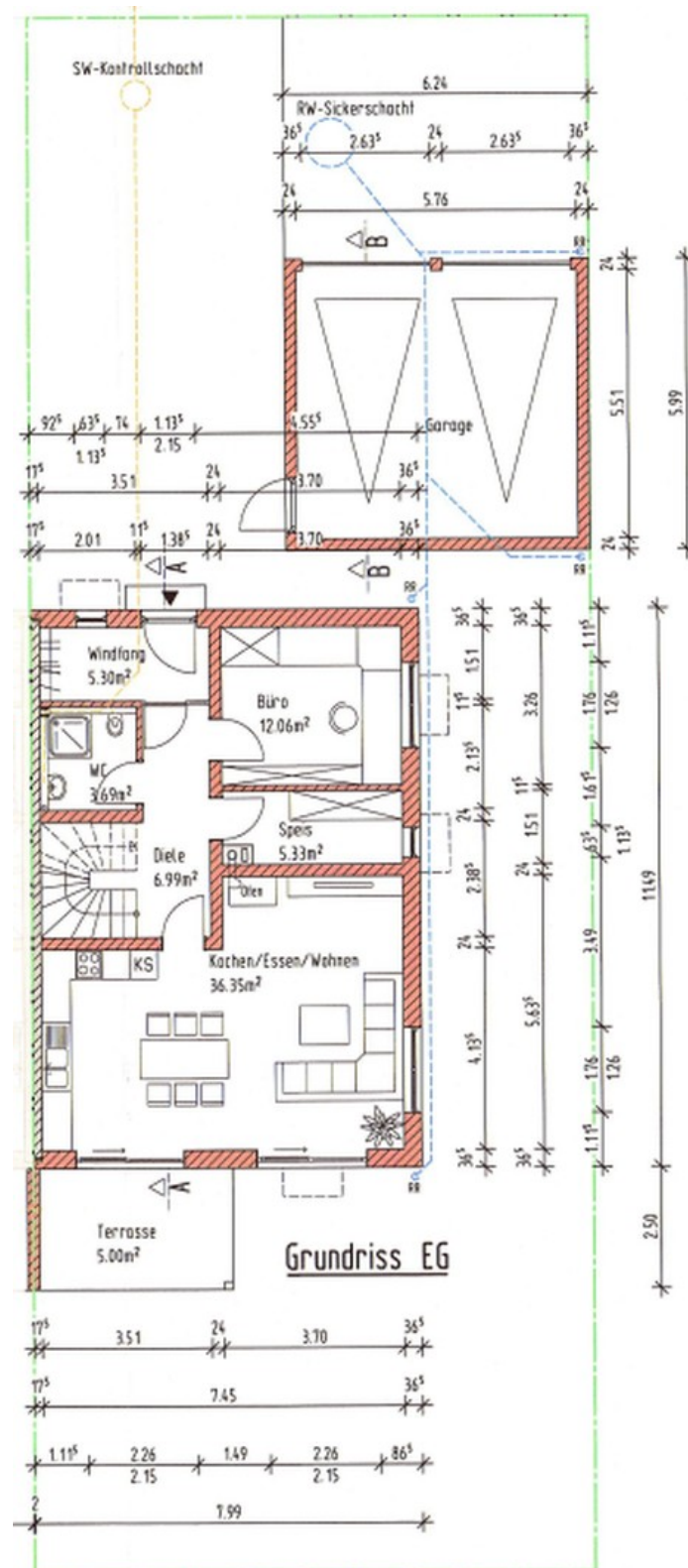
Grundriss (EG)
