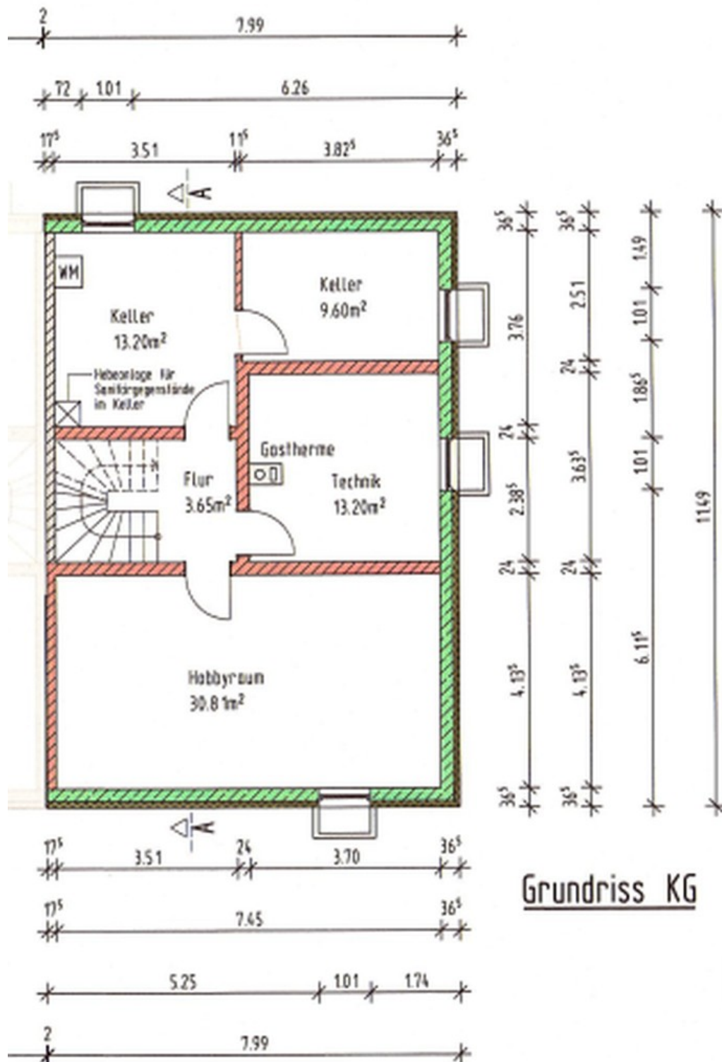
Grundriss (KG)
