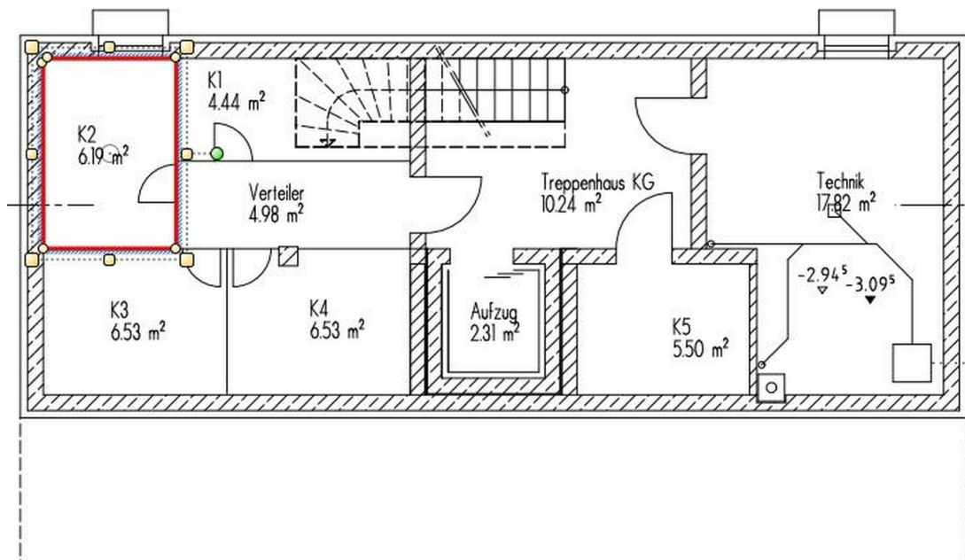
GRUNDRISS KELLERGEOSHOSS
