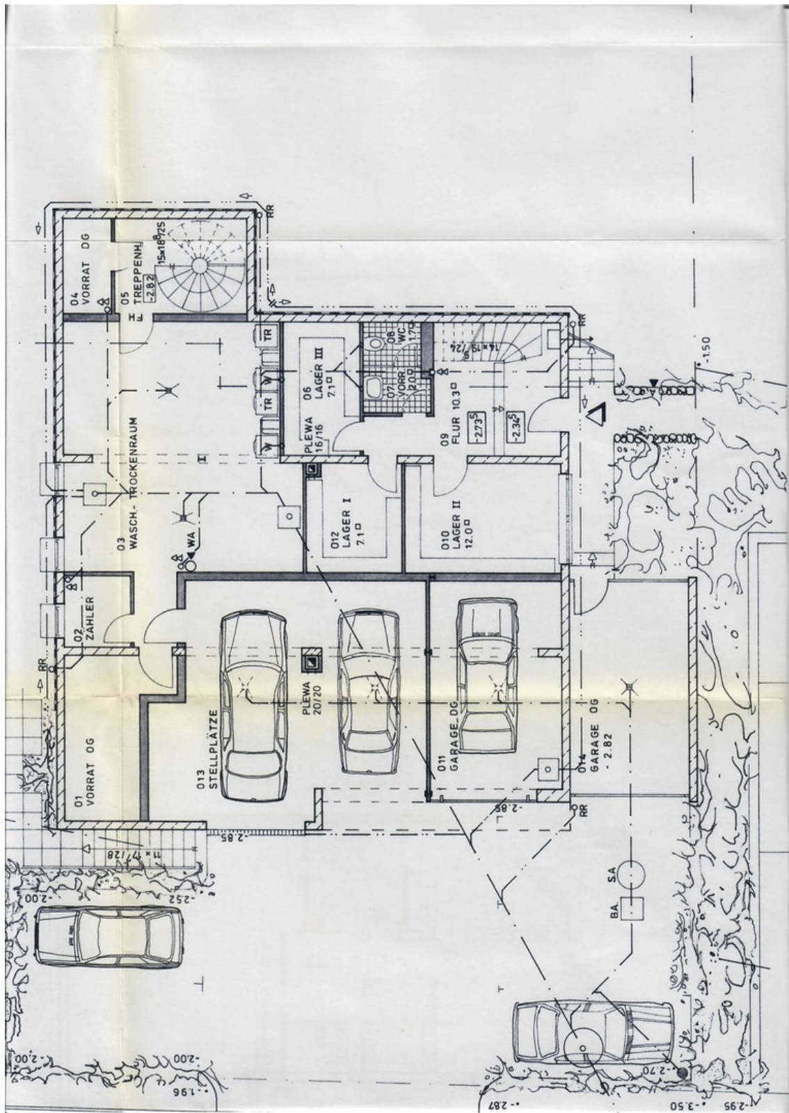
Praxis Kellergeschoss
