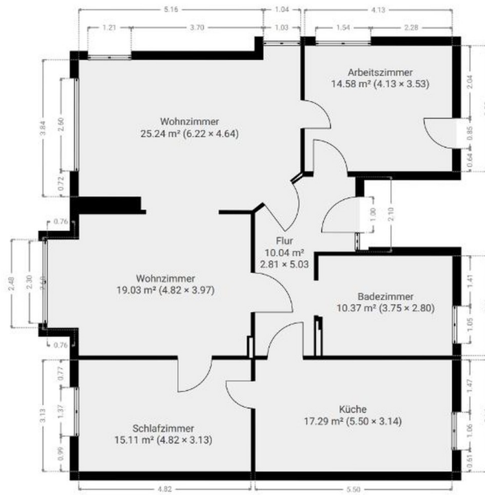
Grundriss
