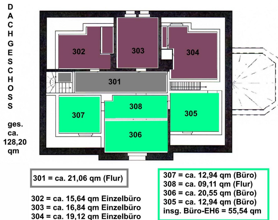
Grundriss DG
