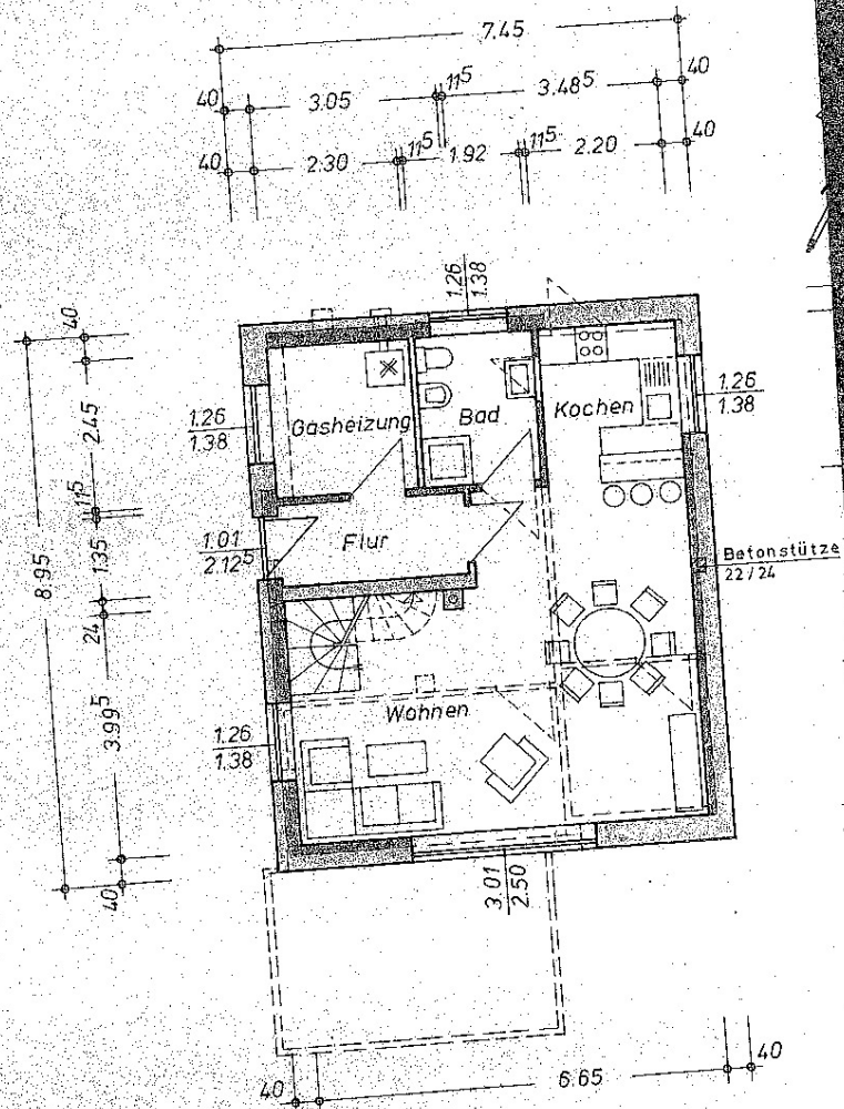
Erdgeschoss
