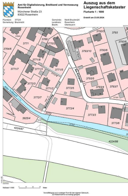
Katasterauszug
