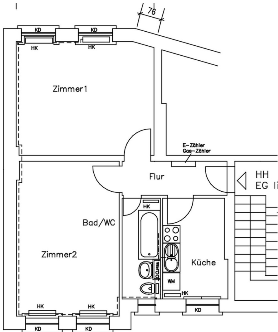
Grundriss
