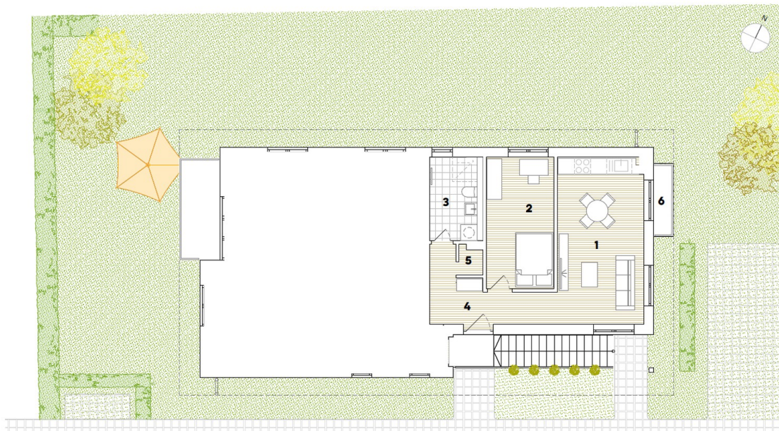
Grundriss
