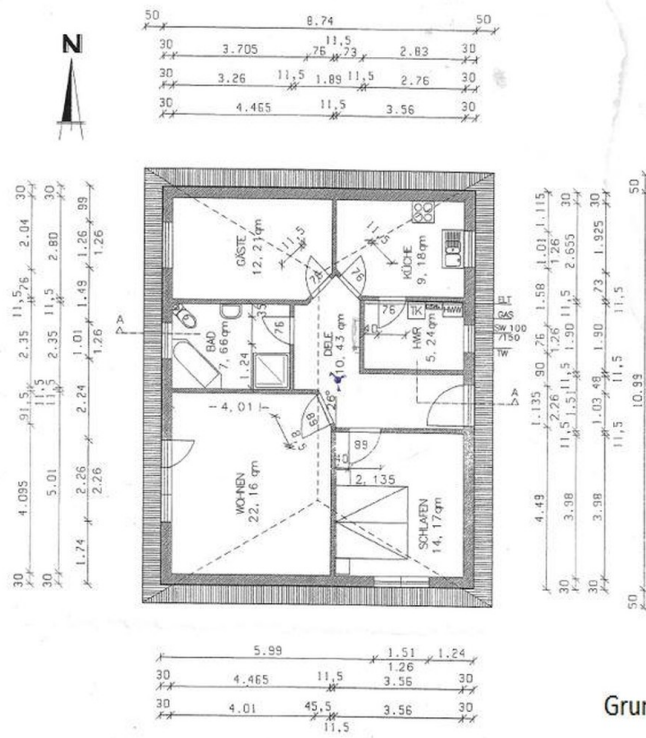
Grundriss
