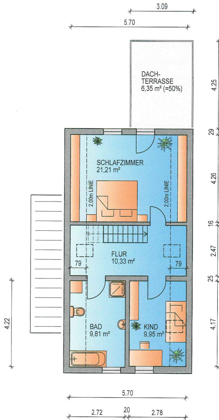
GRUNDRISS DG, M. 1:100
