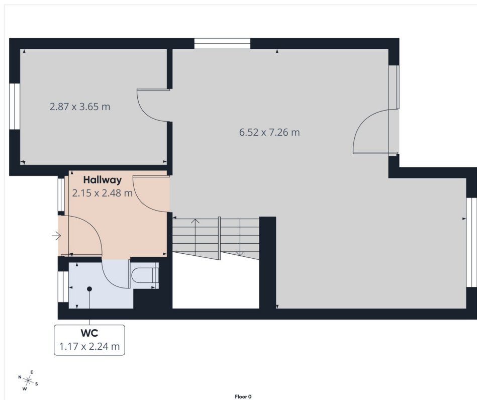
Erdgeschoss
