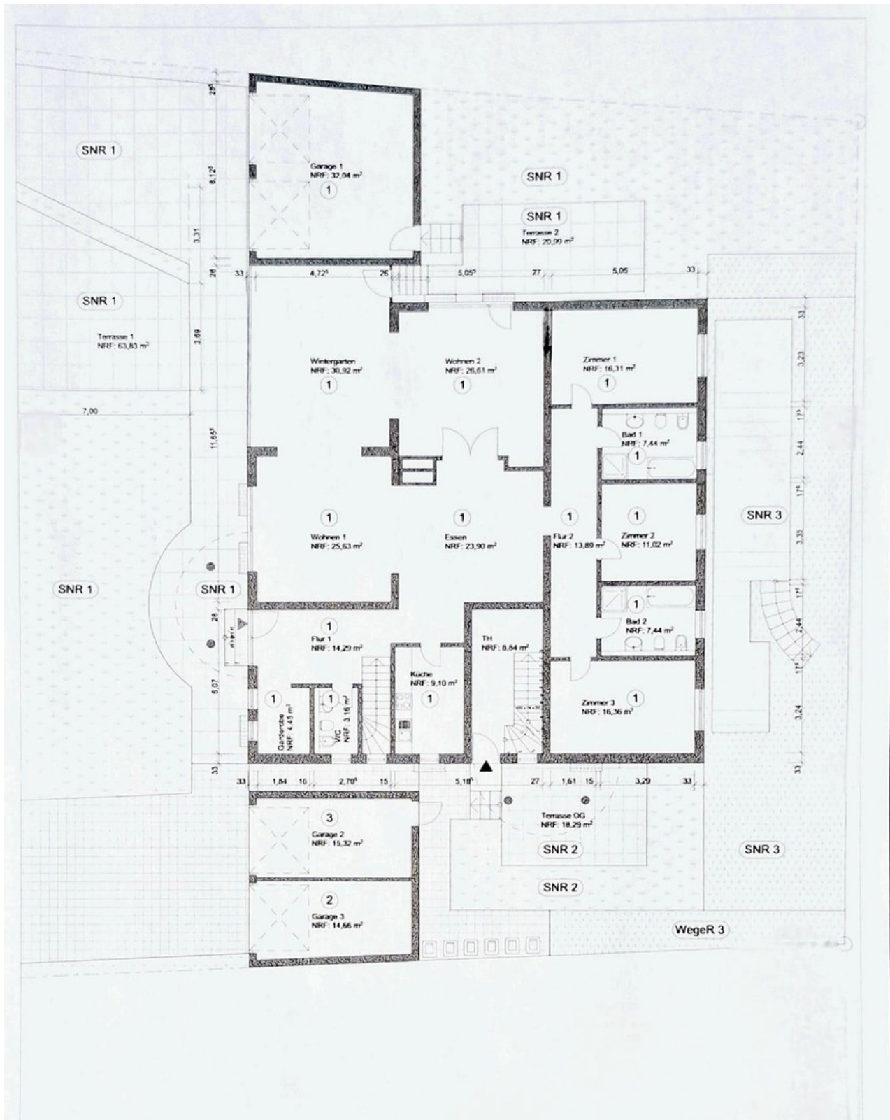
Grundriss EG
