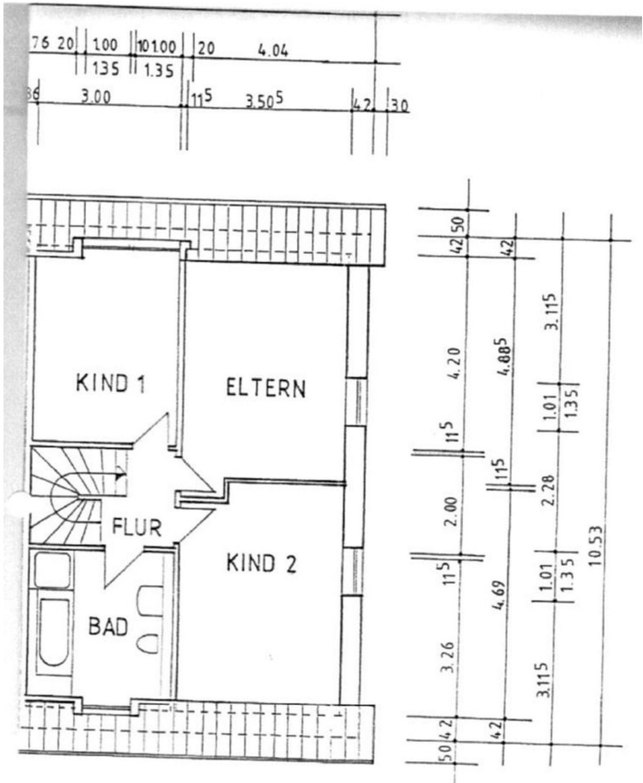
Grundriss DG
