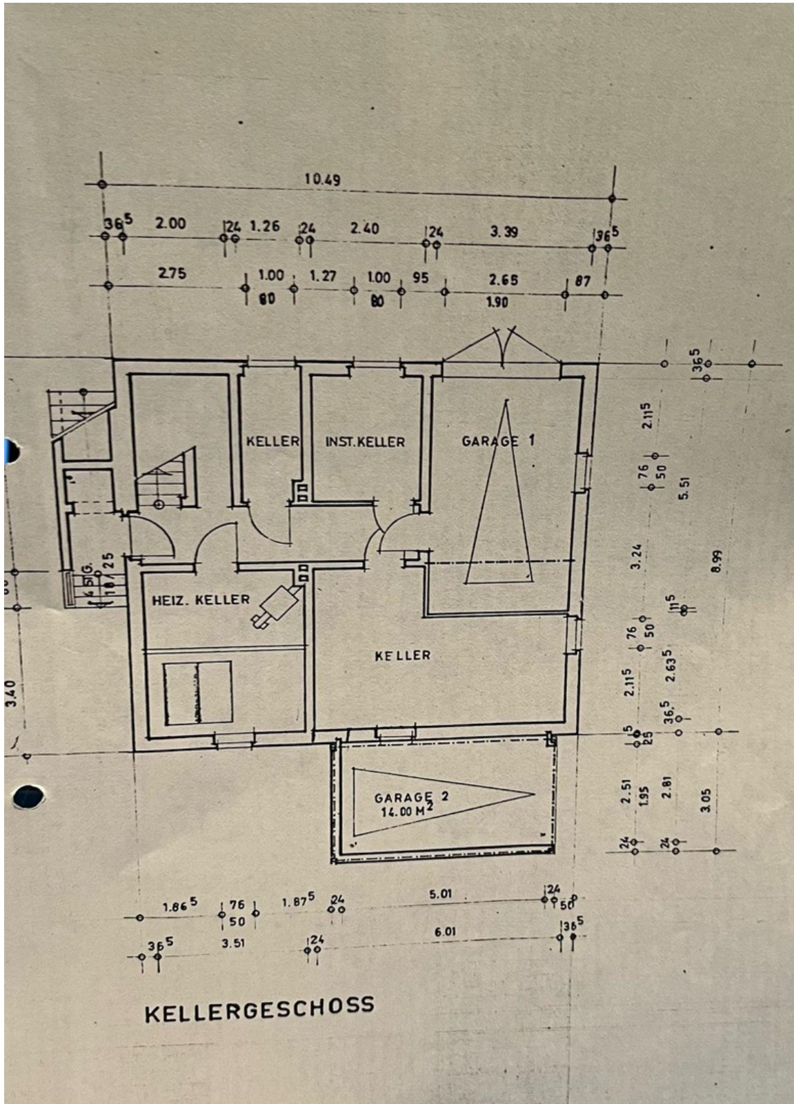
Keller
