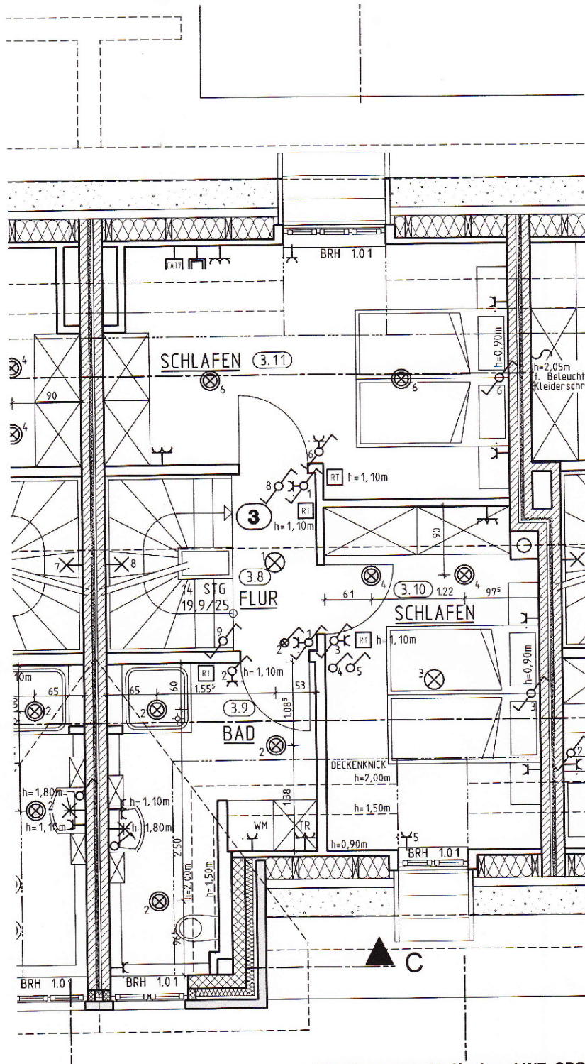
500 Bövergeest 28, Neubau 4 WE, SPO WHG.3_A_1.DG Elektro, 1 : 50, 22.08.2012
