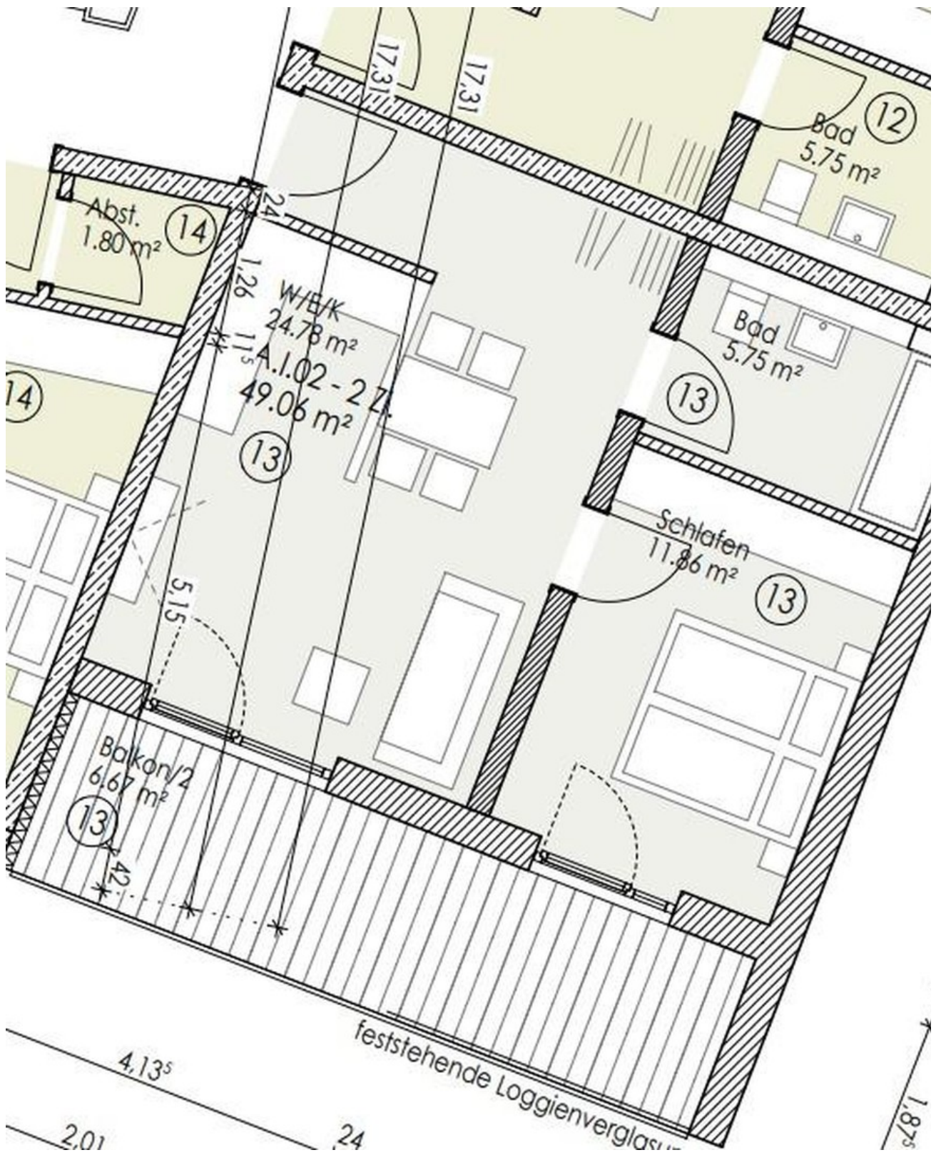
Grundriss Wohnung № 13
