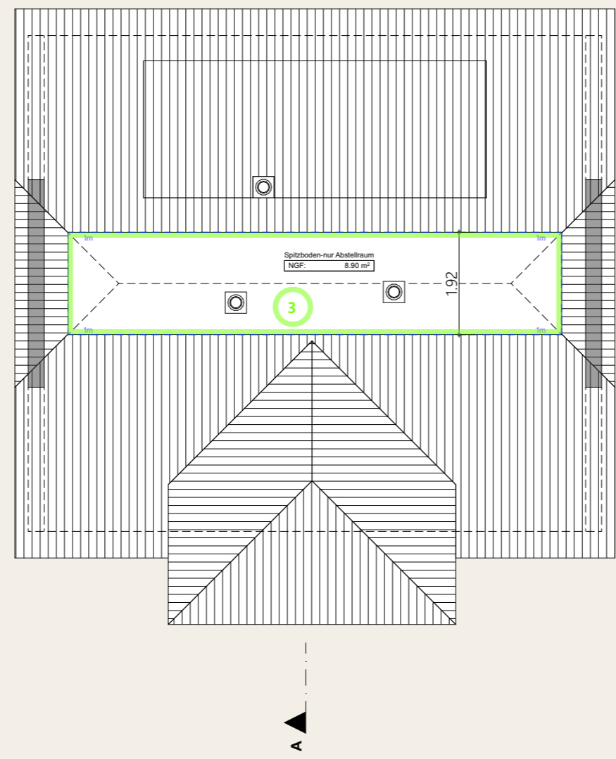
Ansicht Nordwesten
