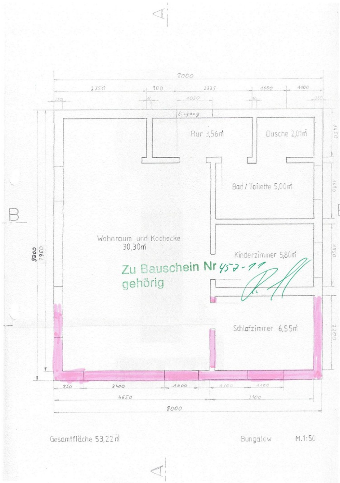
Grundriss
