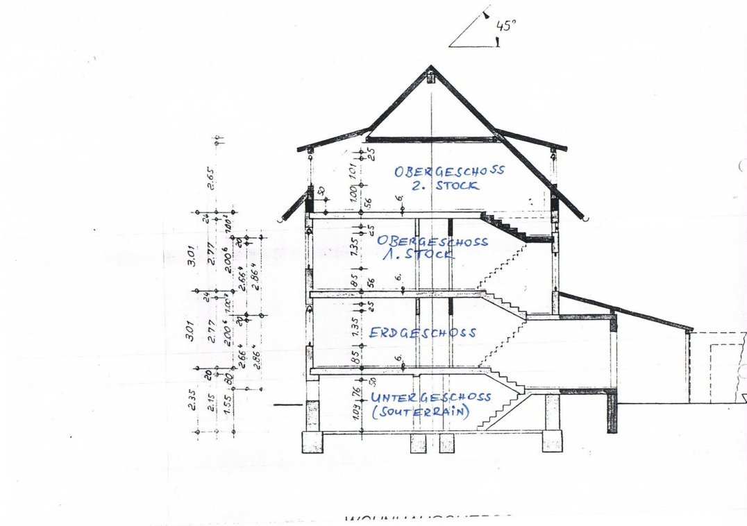
Schnitt
