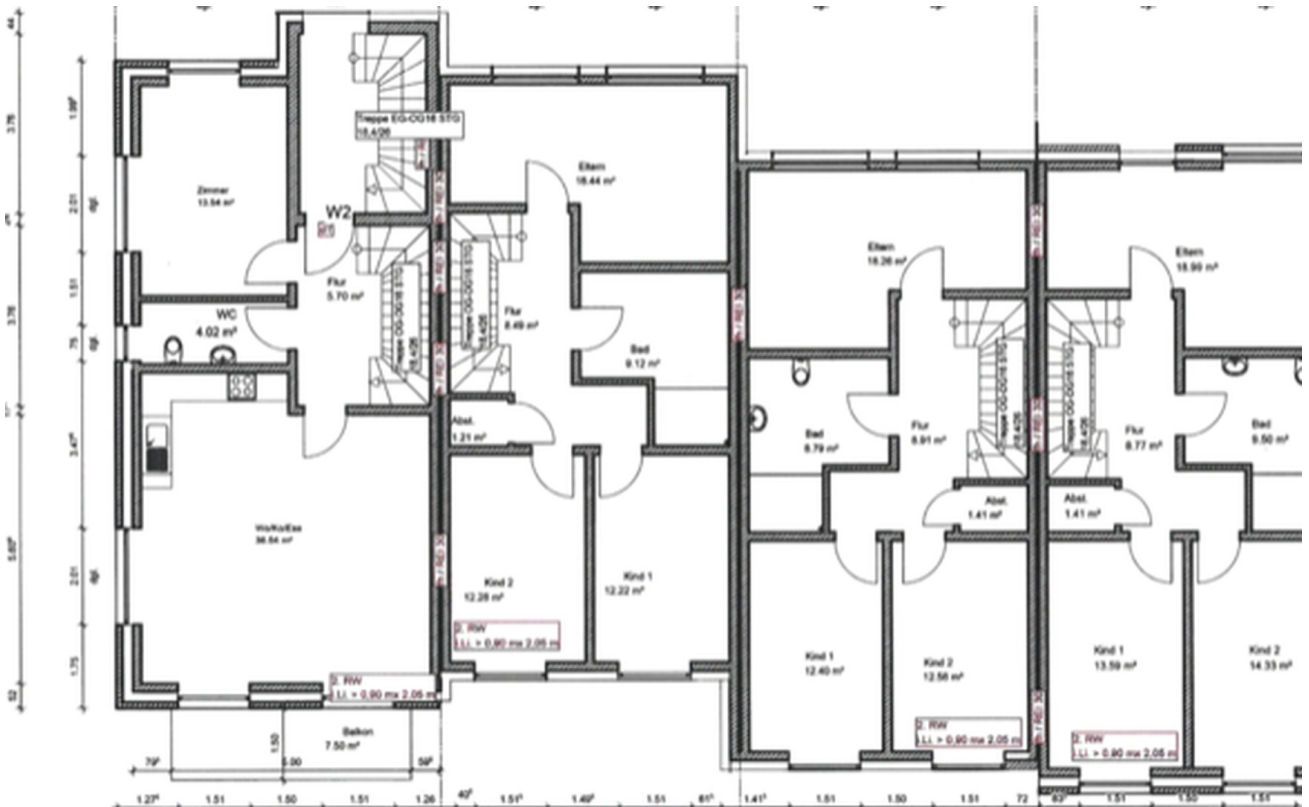
Grundriss 1te OG
