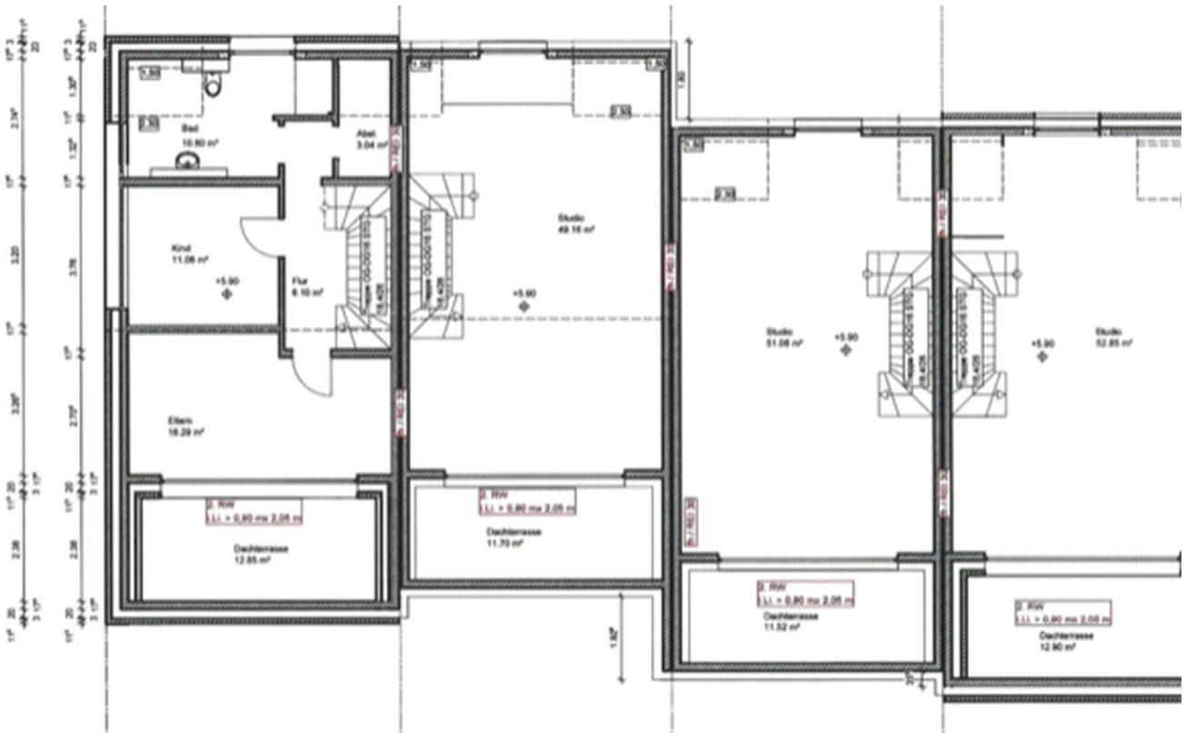
Grundriss 2te OG
