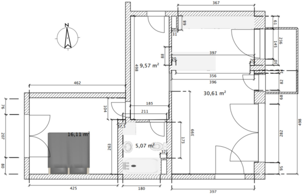
Grundriss
