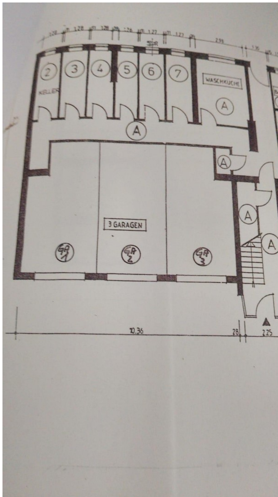
Kellerskizze Whg2
