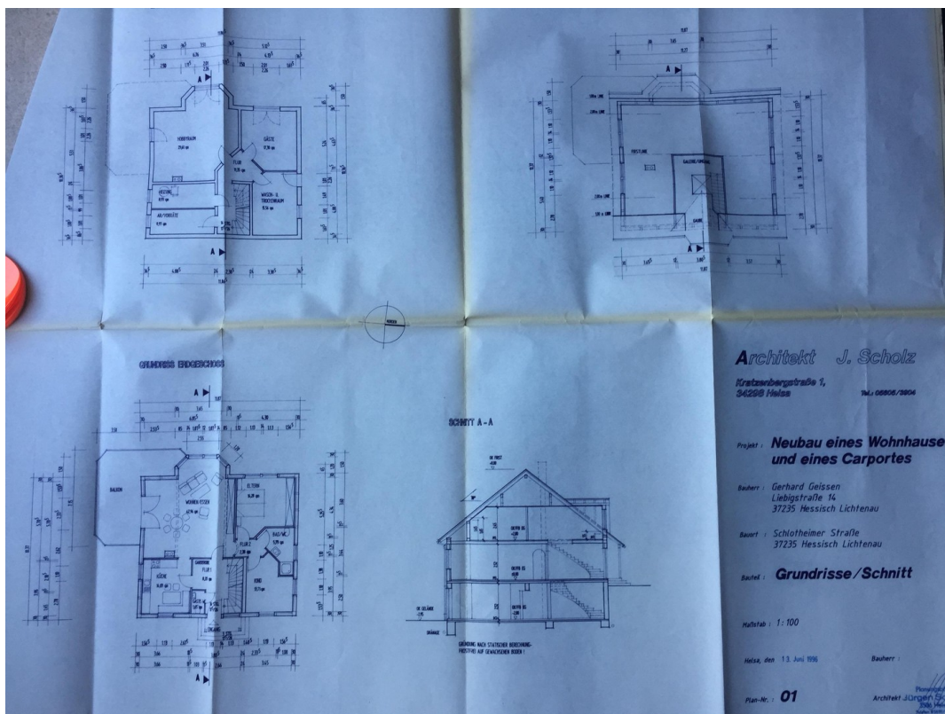
Grundriss und Schnitt
