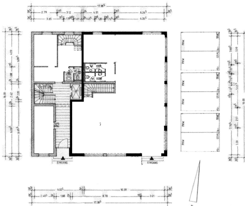
Grundriss EG
