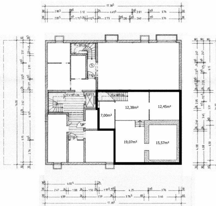
Grundriss KG
