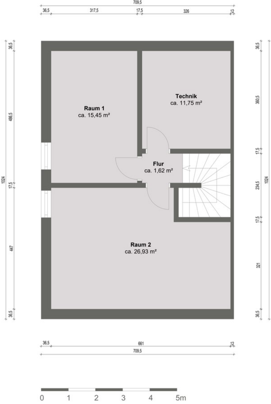
Dachgeschoss
