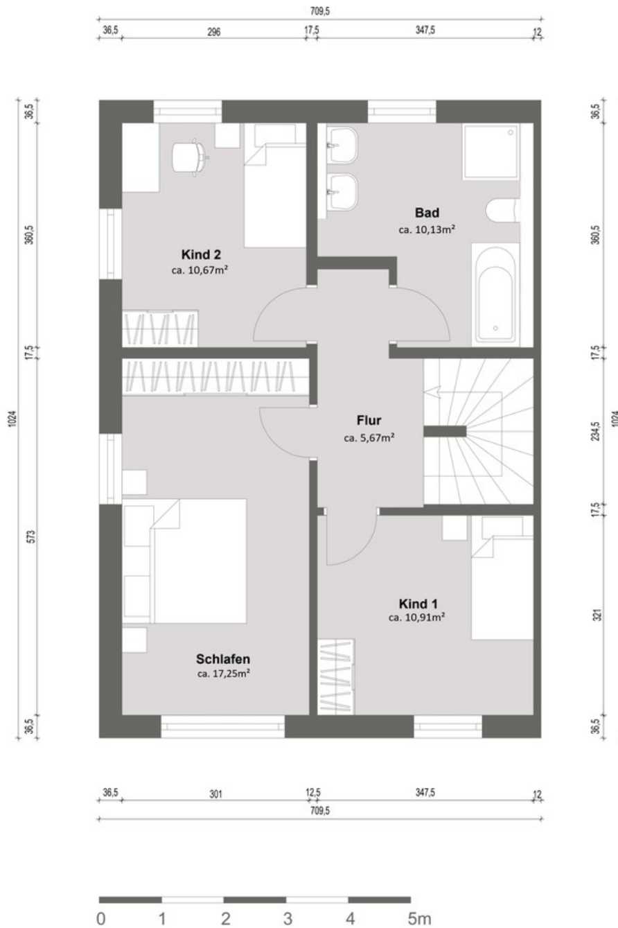
Obergeschoss
