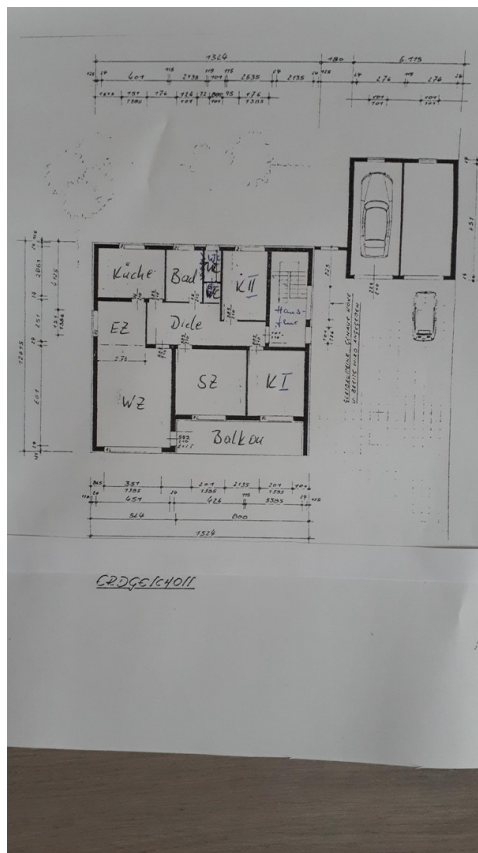
Grundriss EG-Wohnung
