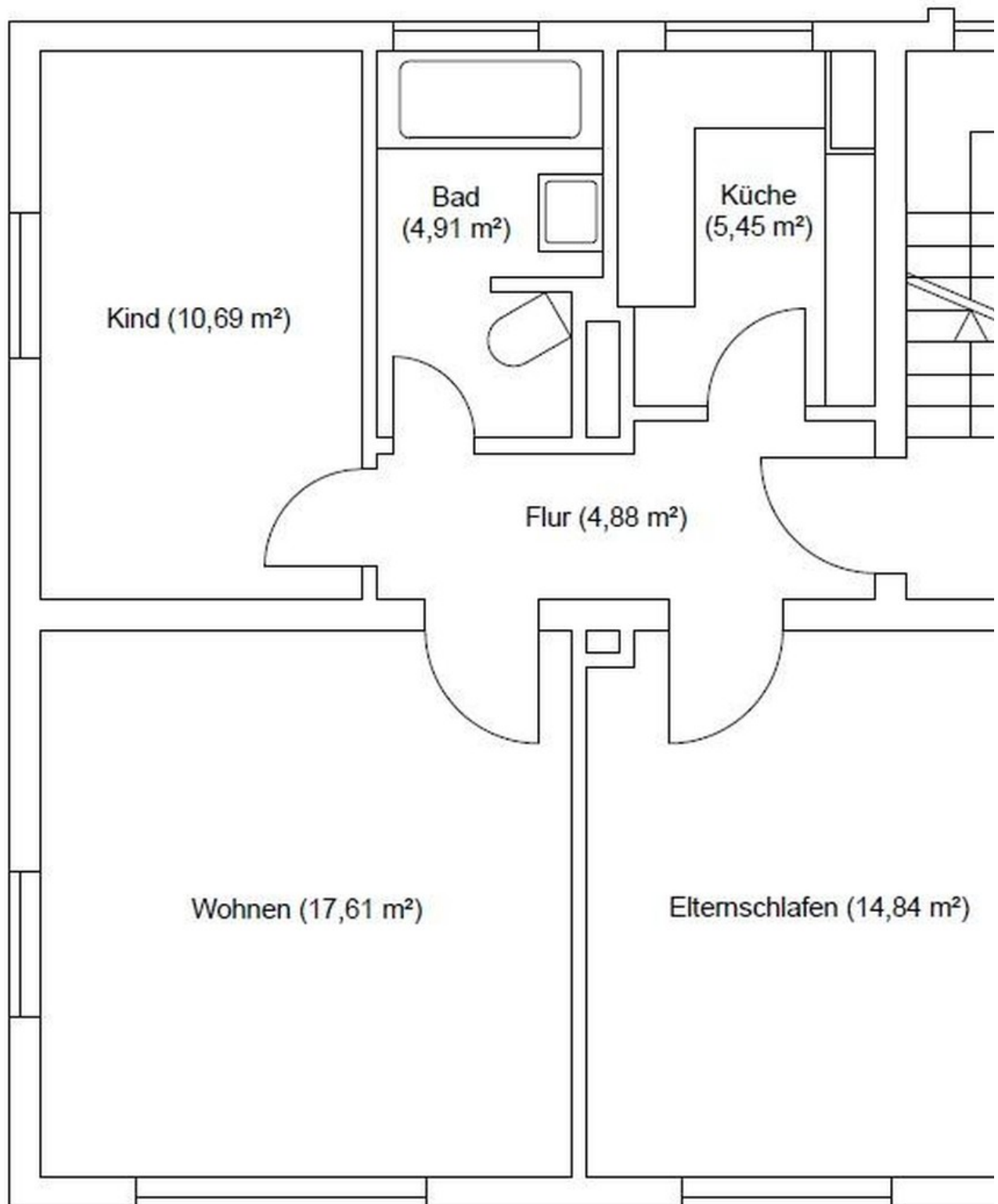
Grundriss rechts
