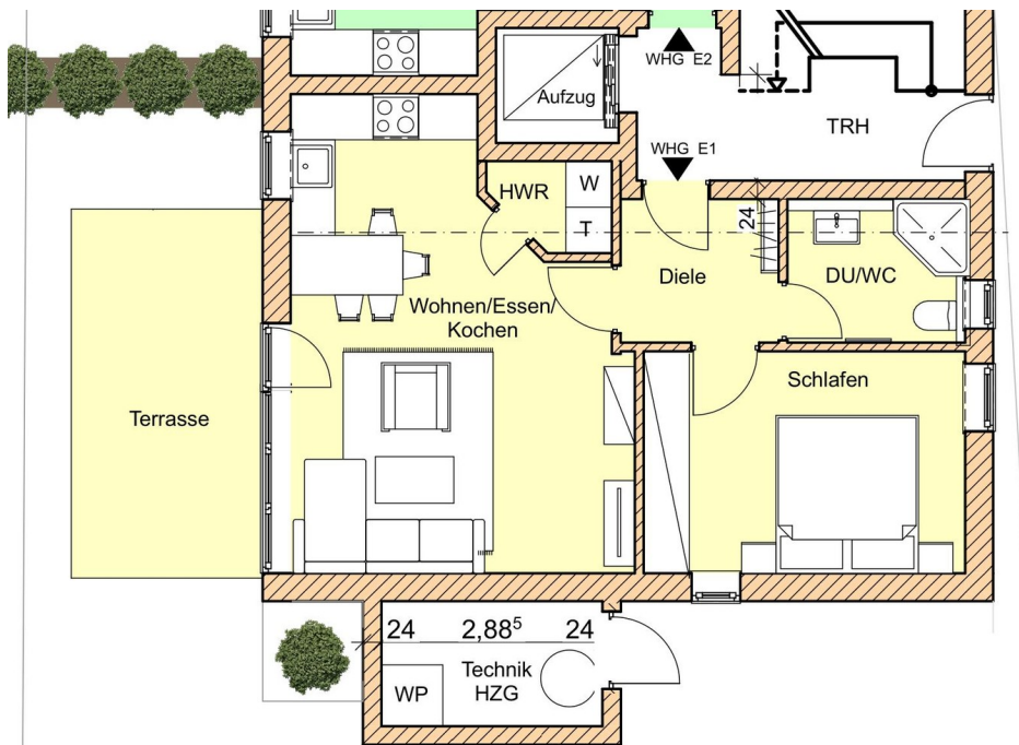
Grundriss EG 1.1
