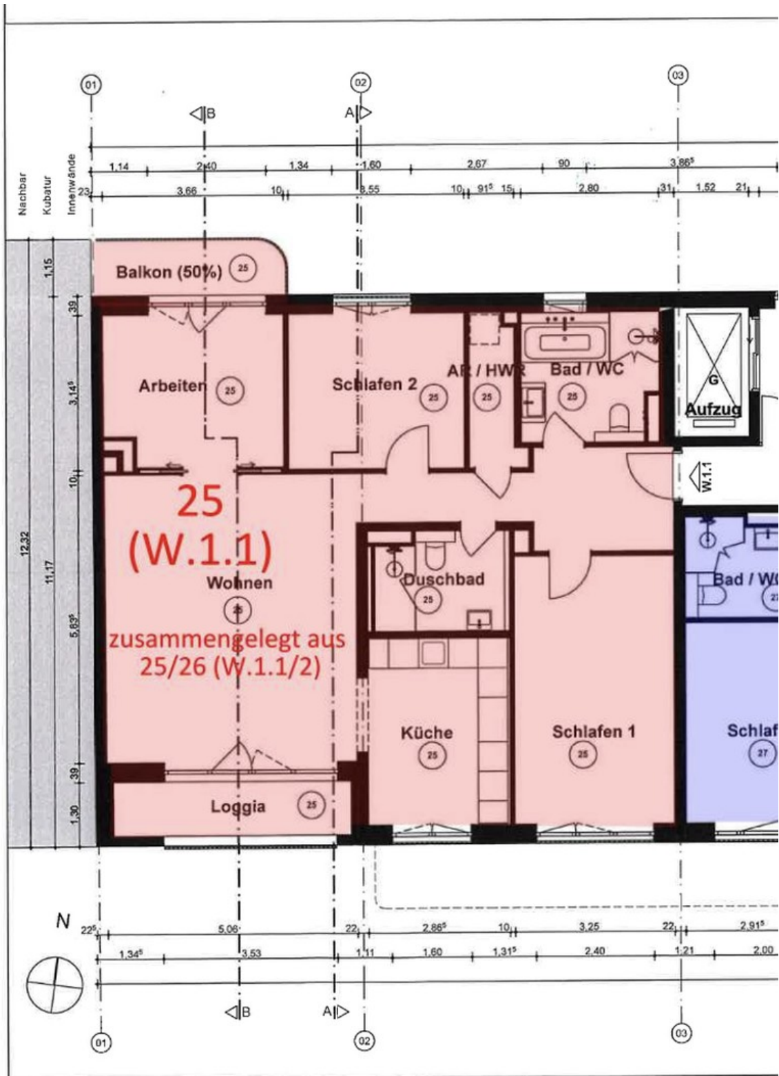
Grundriss
