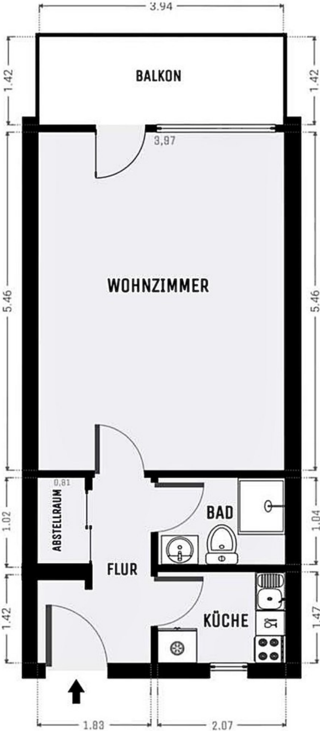
Grundriss
